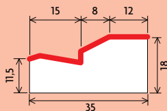
Bordure AC1
